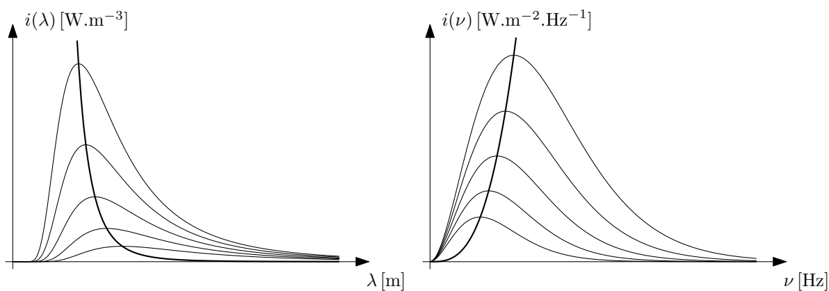
(a) Spektrální hustoty i(\lambda, T) a jejich maxima.
