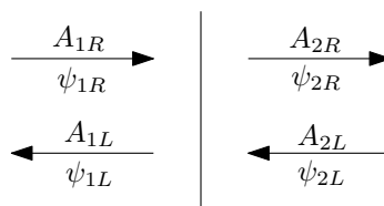
Obrázek 4.8: Rozhraní mezi dvěma prostředími. V obou prostředích se šíří postupné vlny oběma směry označené \psi_{1R} (vlna v prvním prostředí postupující doprava), \psi_{1L} (vlna v prvním prostředí postupující doleva), \psi_{2R} a \psi_{2L} (analogicky v druhém prostředí). Jejich amplitudy jsou označené A_{1R} , A_{1L} , A_{2R} a A_{2L} .
