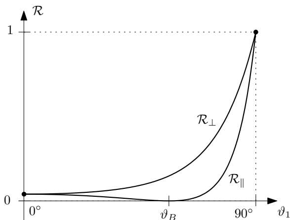
(c) Odrazivosti pro odraz na opticky hustším prostředí, tzn. situace pro n_1 < n_2 .
