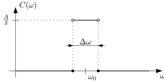
Obrázek 3.10: Obdélníkové spektrum.
