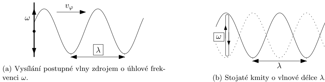
Obrázek 3.2: Disperzní vztah udává vztah mezi úhlovou frekvencí \omega a vlnovým číslem k = \frac{2\pi}{\lambda} (a tedy vlnovou délkou \lambda ).
