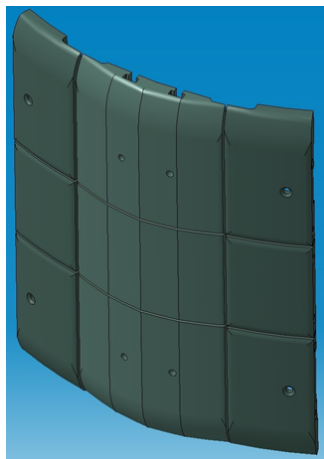
Obrázek 4.1: 3D model speciální grafitové dlaždice pro limiter tokamaku COMPASS [15].
