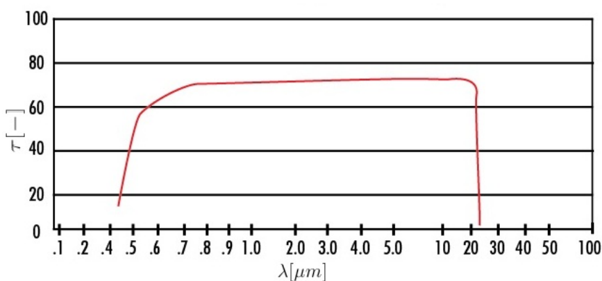
Obrázek 2.2: Transmittance ZnSe sklíčka v závislosti na vlnové délce \lambda . [2]
