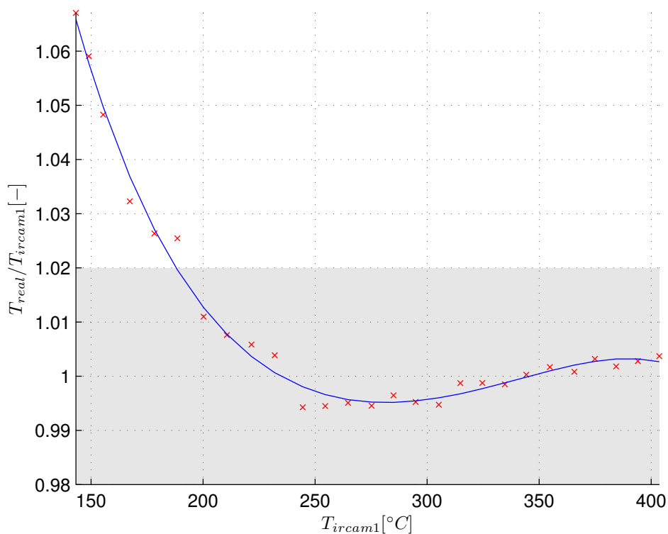
Obrázek 3.5: Kalibrační funkce pro kameru bez přidaných optických prvků a pro teplotní rozsah 150...900 °C. Červeně naměřená data, modře nafitovaný polynom f_{900} , šedě vyznačena přesnost udávaná výrobcem.
