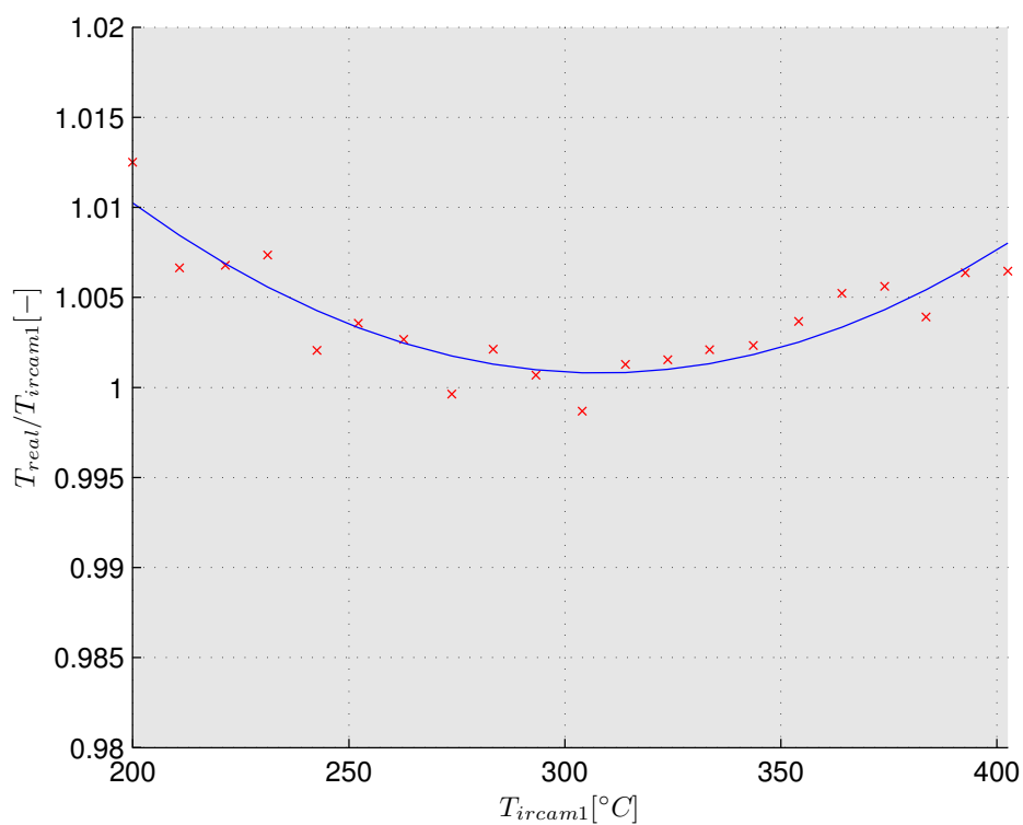
Obrázek 3.6: Kalibrační funkce pro kameru bez přidaných optických prvků a pro teplotní rozsah 200...1500 °C. Červeně naměřená data, modře nafitovaný polynom f_{1500} , šedě vyznačena přesnost udávaná výrobcem.
