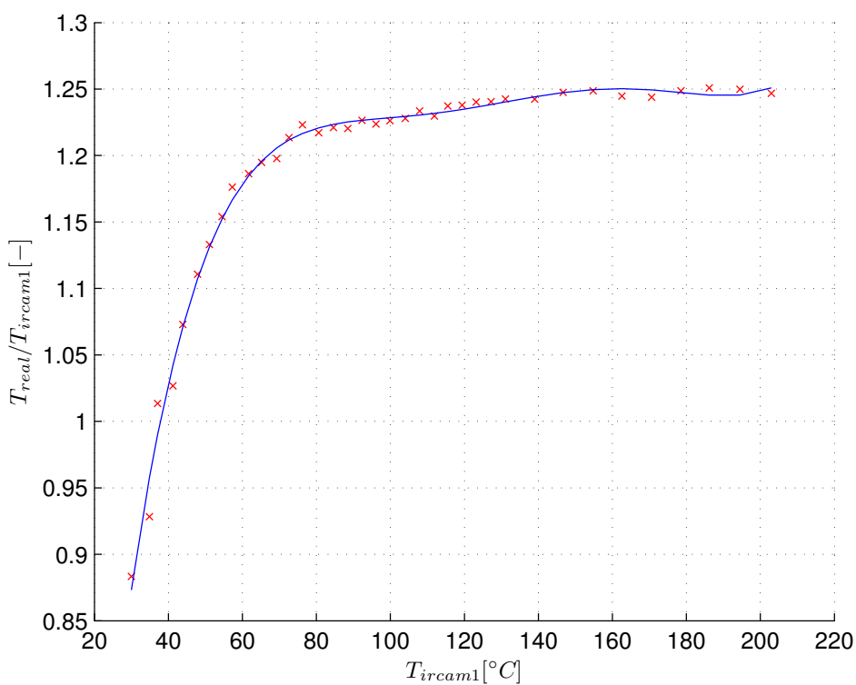
Obrázek 3.8: Kalibrační funkce pro kameru se ZnSe sklíčkem a pro teplotní rozsah 0...250 °C. Červeně naměřená data, modře naitovaný polynom f_{ZnSe250} .
