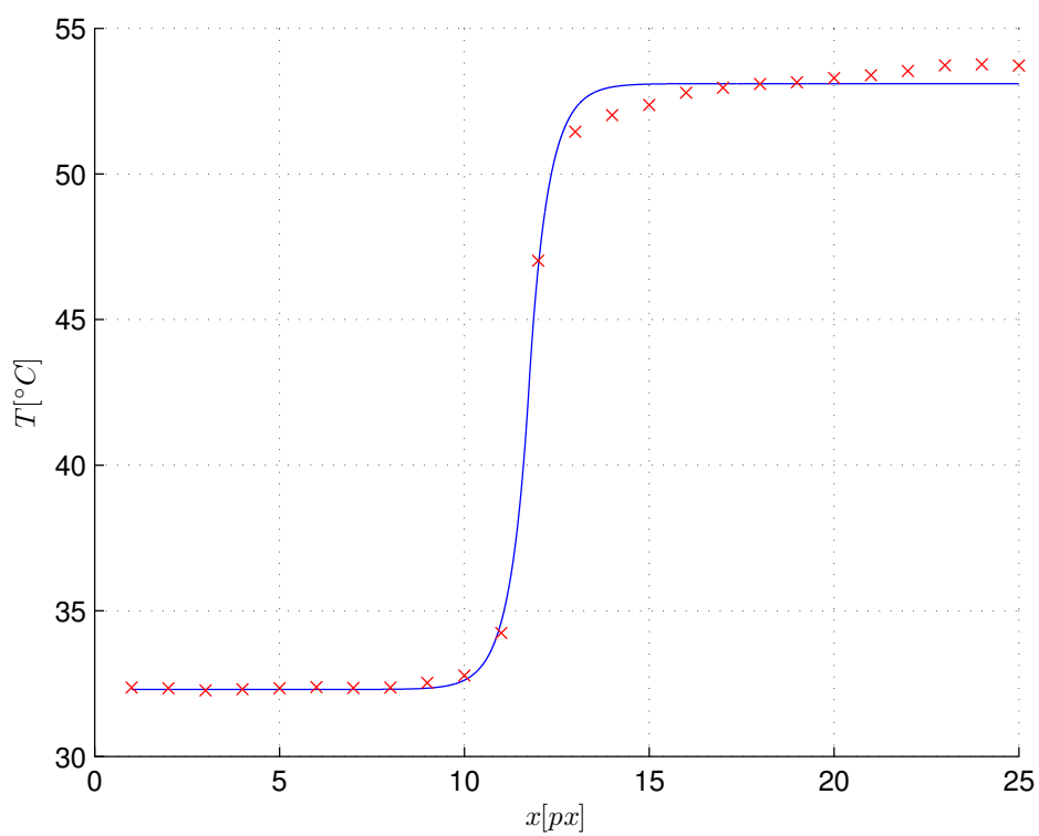
Obrázek 3.17: Červeně naměřená data pro vertikální skok teploty T proložená funkcí f (modře)
