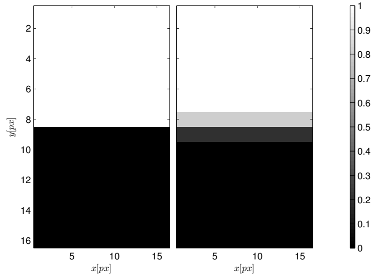
Obrázek 3.19: Vliv PSF na obraz. Vlevo testovací skoková změna signálu. Vpravo obraz po rozostření skoku funkcí PSF z tabulky 3.2.
