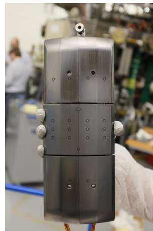
Obrázek 4.2: Speciální grafitová dlaždice pro limiter tokamaku COMPASS. [15]
