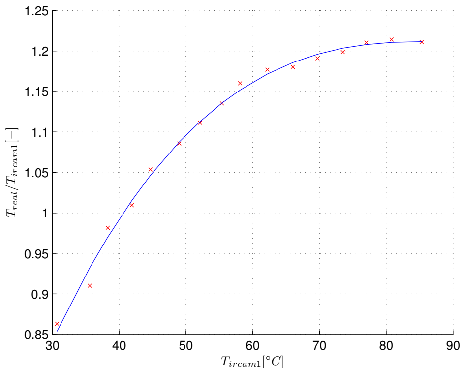
Obrázek 3.7: Kalibrační funkce pro kameru se ZnSe sklíčkem a pro teplotní rozsah -20...100 °C. Červeně naměřená data, modře naitovaný polynom f_{ZnSe100} .
