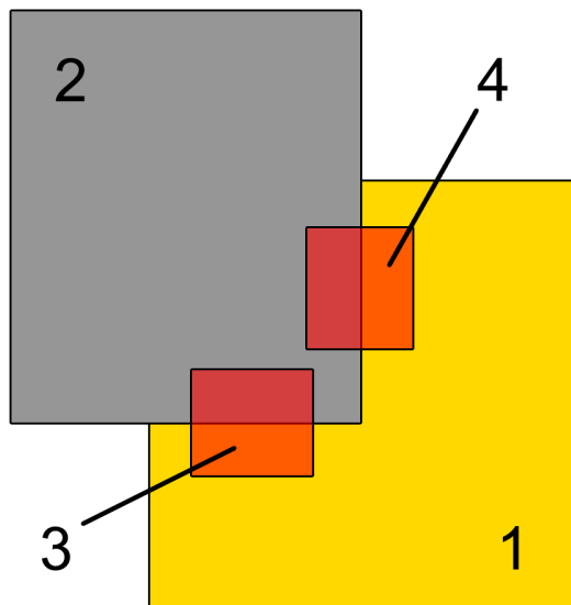
Obrázek 3.14: Schéma měření zkreslení skokové změny teploty. 1 – zahřáté těleso, 2 – clona, 3 – snímaná oblast pro vertikální změnu teploty, 4 – snímaná oblast pro horizontální změnu teploty
