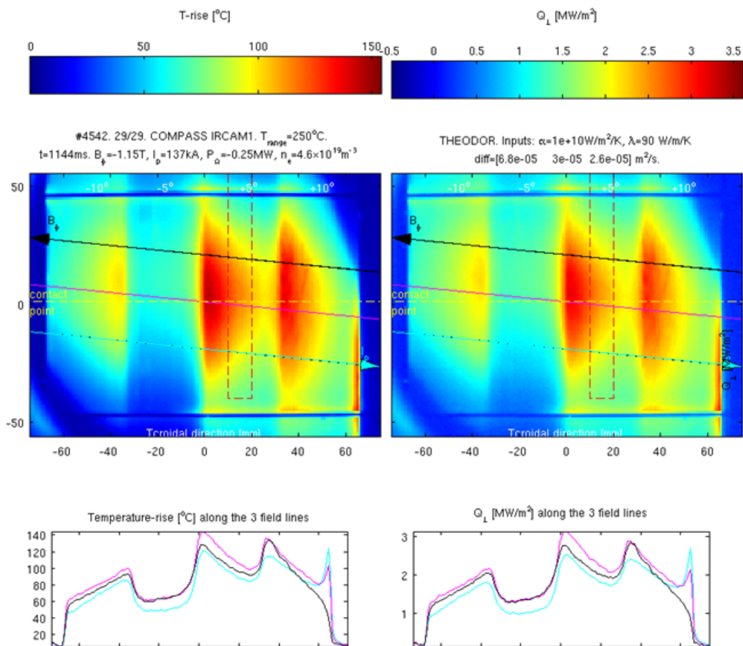
Obrázek 4.3: Snímek z IR kamery na tokamaku COMPASS. Levý graf ukazuje teploty na dlaždici limiteru, pravý graf tepelné toky vypočtené pomocí kódu THEODOR. Černá šipka označuje směr magnetického pole, bledě modrá šipka směr proudu v plazmatu. Grafy ve spodní části obrázku obsahují průběh teploty, resp. tepelného toku, podél tří magnetických siločar.
