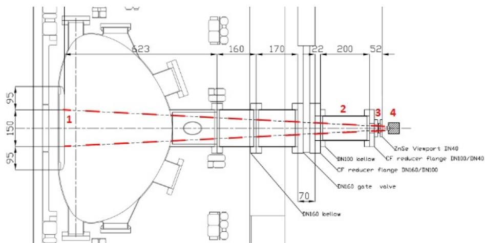
Obrázek 2.1: Schéma umístění IR kamery na tokamaku COMPASS, boční pohled. 1 – pozorované cihličky vnitřní stěny, 2 – vlnovec, 3 – ZnSe sklíčko, 4 – IR kamera. Převzato z [15].
