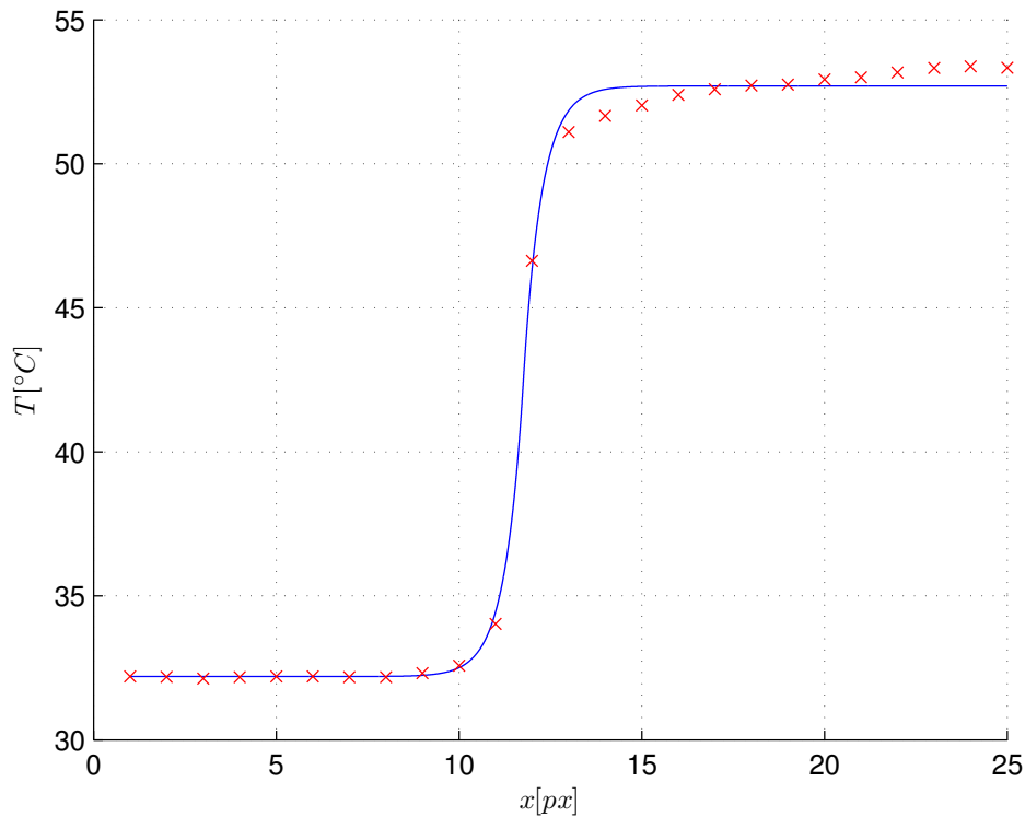
Obrázek 3.18: Červeně naměřená data pro vertikální skok teploty T proložená funkcí f (modře)
